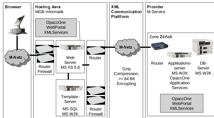
Abb. 11.3: Hardware-Architektur
